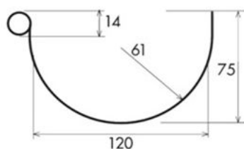
Sección GRN125
