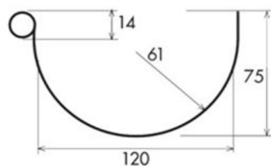
Sección GRN125
