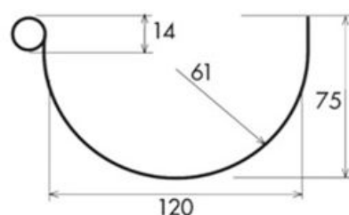
Sección GRN125
